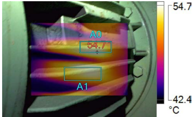
IR005250.IS2-No2 Aux Blower
