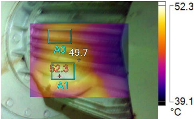
IR005252.IS2-No2 Aux Blower
