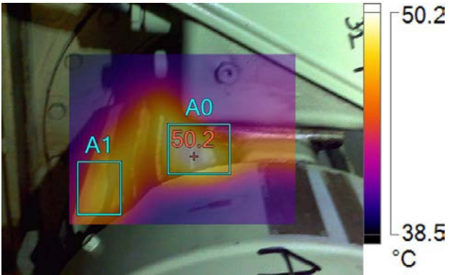
IR005248.IS2-No2 Aux Blower
