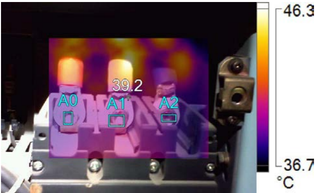
IR005149.IS2-No2 Main LO pump
