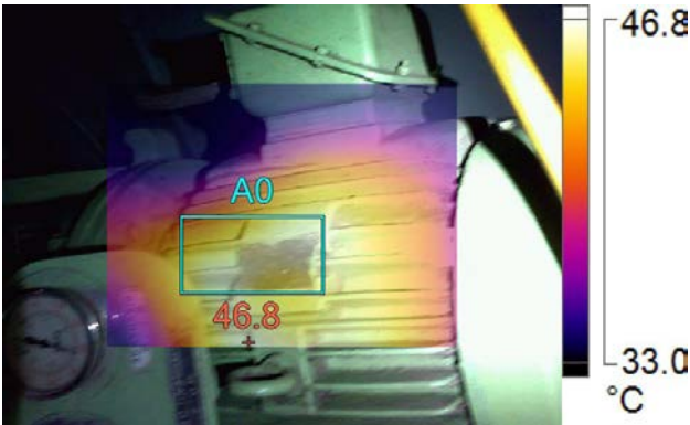
IR005241.IS2-No2 Crosshead LO pump 12/3/2016 2:51:00 PM
