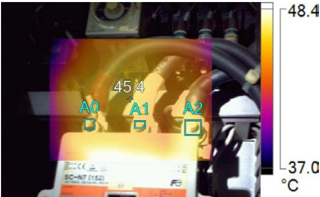
IR005153.IS2-No2 Main LO pump
