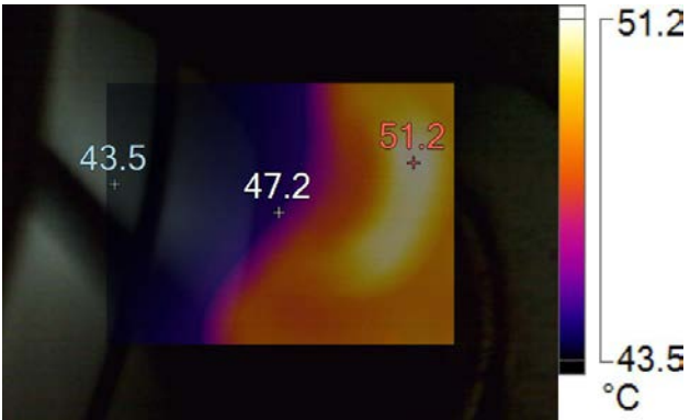
IR005244.IS2-No2 Crosshead LO pump 12/3/2016 2:52:42 PM
