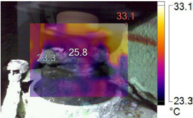
IR005198.IS2-FWG Ejector pump 12/3/2016 1:18:43 PM
