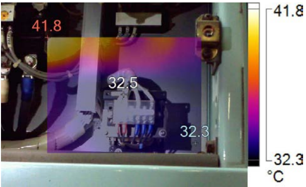
IR005152.IS2-No2 Main LO pump
