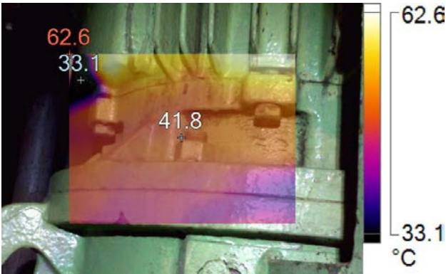
IR005243.IS2-No2 Crosshead LO pump 12/3/2016 2:52:07 PM
