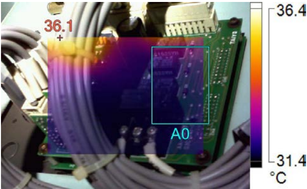
IR005237.IS2-No2 Crosshead LO pump 12/3/2016 2:48:58 PM
