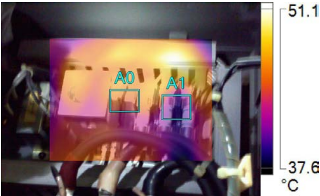
IR005154.IS2-No2 Main LO pump
