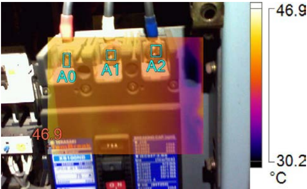
IR005231.IS2-No2 Crosshead LO pump 12/3/2016 2:47:06 PM
