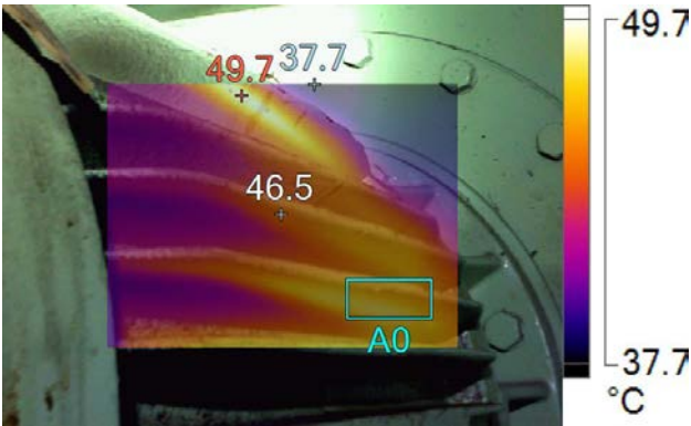
IR005251.IS2-No2 Aux Blower
